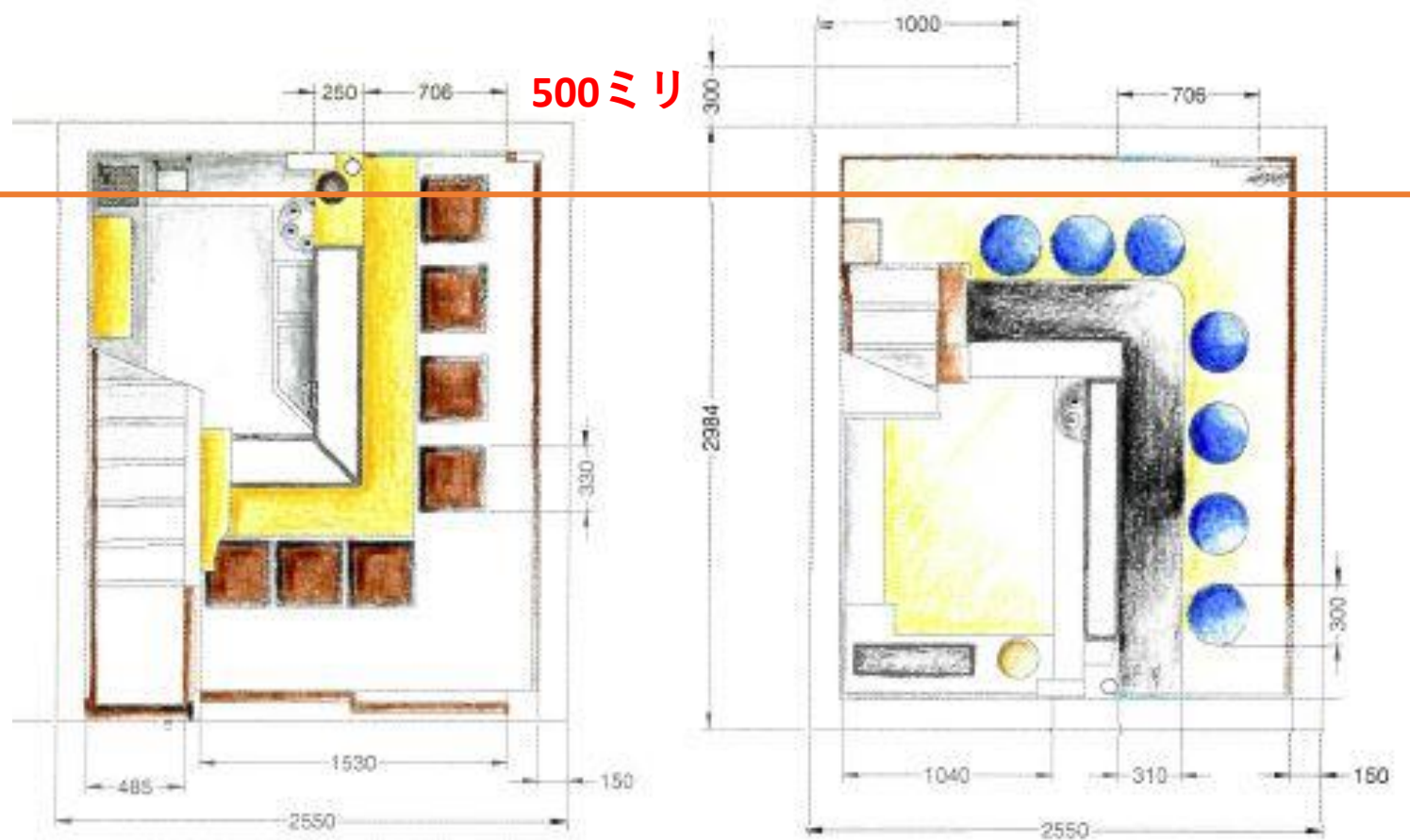
1階平面図
