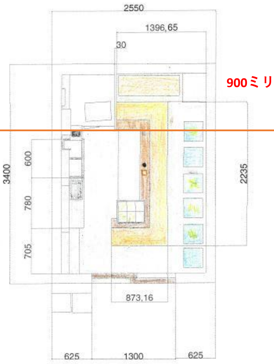
平面図
