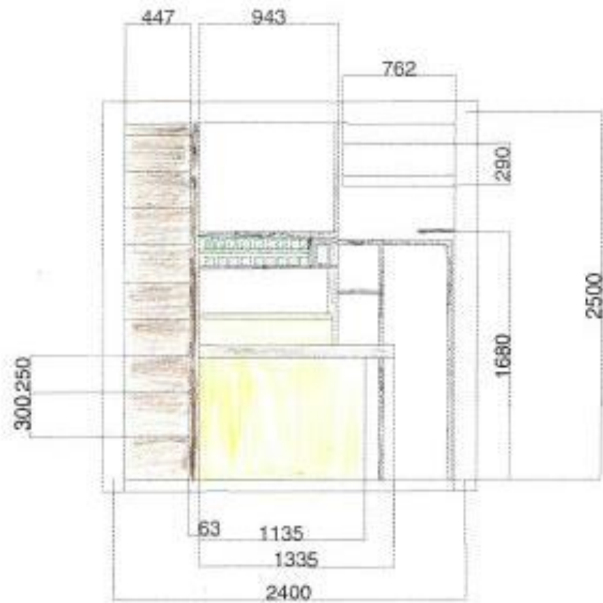
断面図
