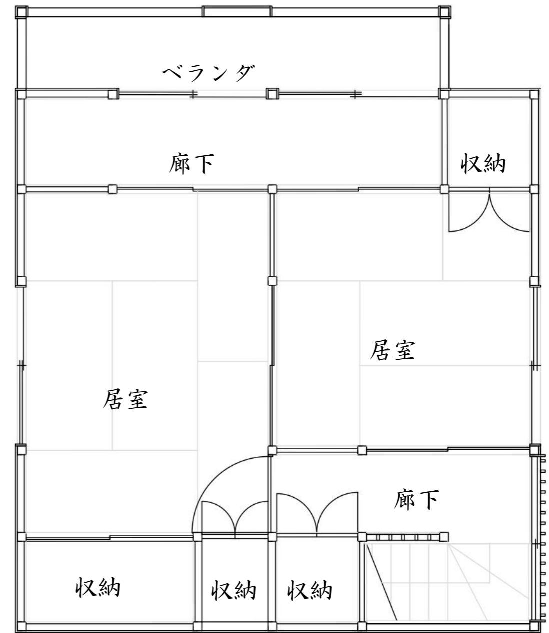
現在 1/40 2階平面図
