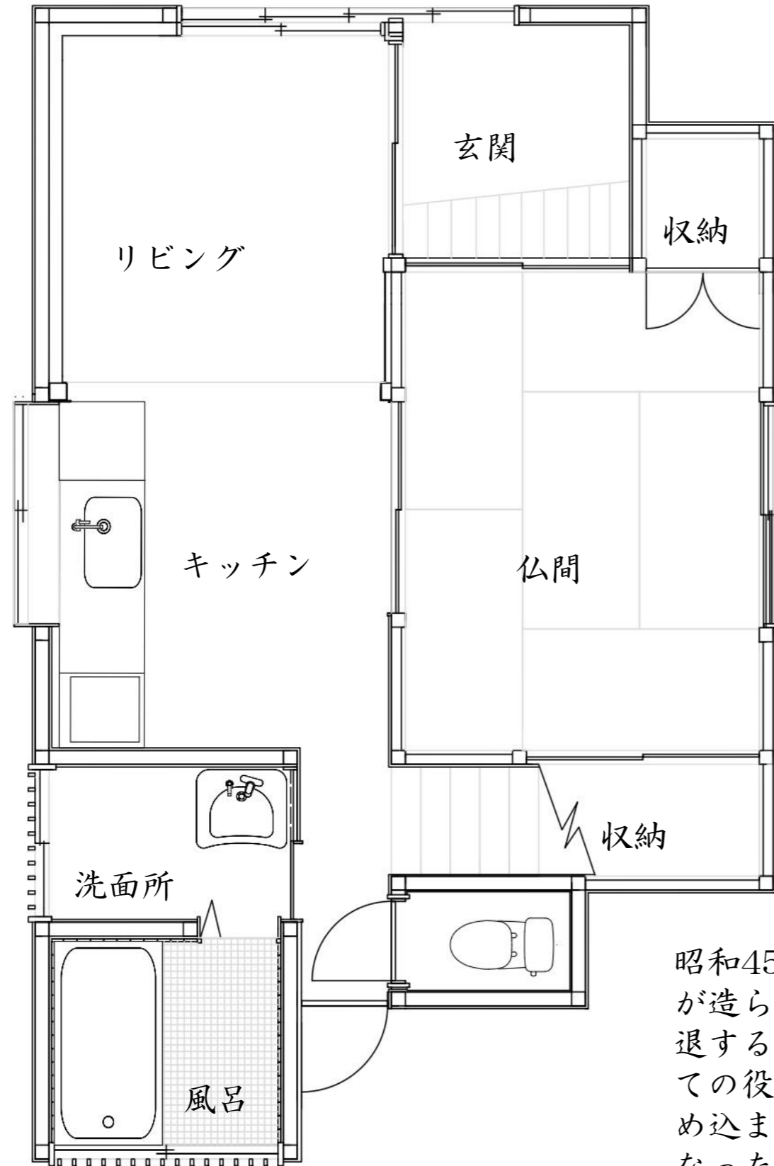
現在 1/40 1階平面図
