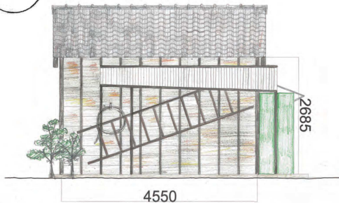
西侧立面
